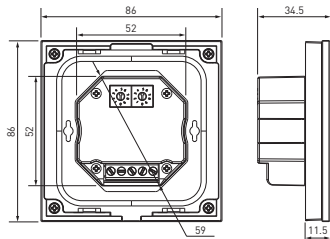
Рис. 1. Габаритный чертеж
